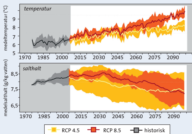
Temperatur och salthalt i Östersjön enligt två klimascenarier
