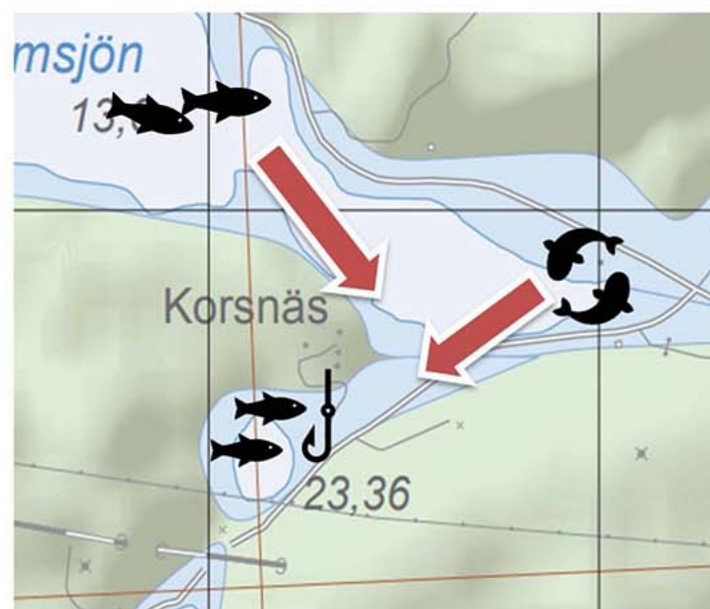
Figur 2. Rekonstruerad strandlinjekarta över Korsnäs för ca 4500 år sedan.
