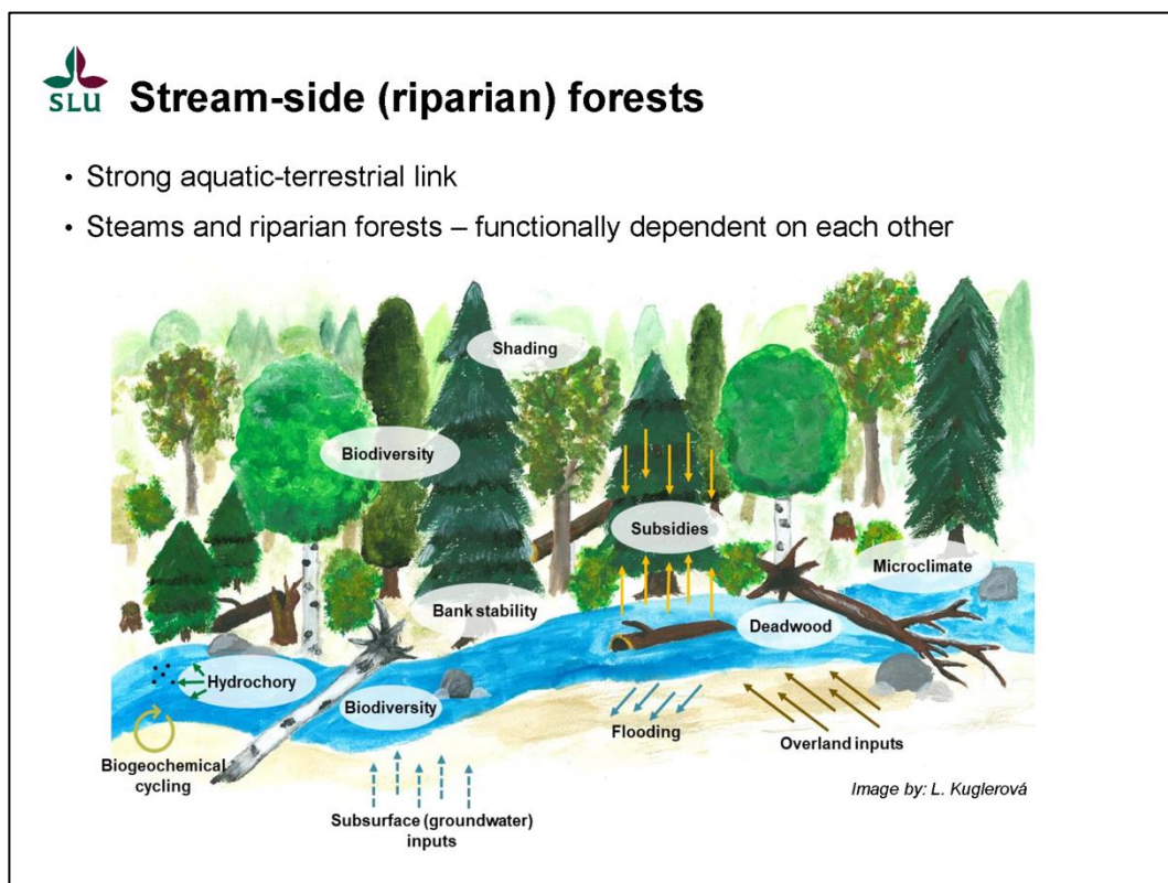
Figur 8. I strandzonen binds skogs- och vattenmiljöerna ihop av en rad processer, som gör att miljöerna påverkar varandra.
