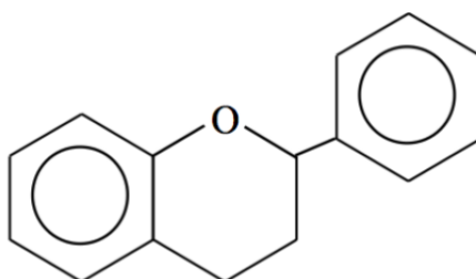
Figur 1: En generell strukturformel för gruppen flavonoider.
